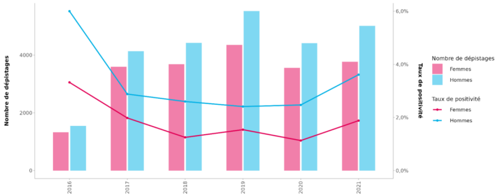
Figure 20 : Courbe d'évolution du nombre de dépistage et taux de positivité des infections à gonocoque en Cegidd, Normandie, 2016-2021
